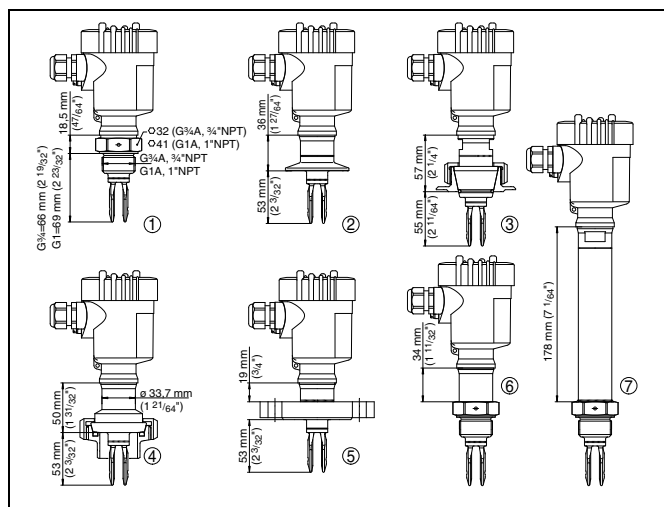
Fig. 51: VEGASWING 61
