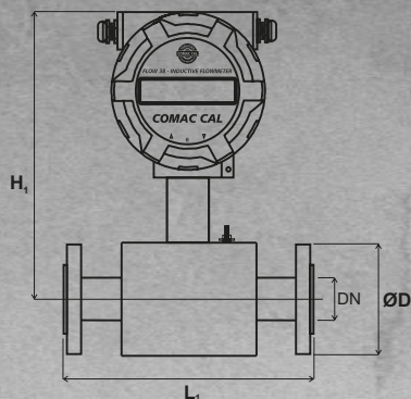
FLANGE (EN 1092)
