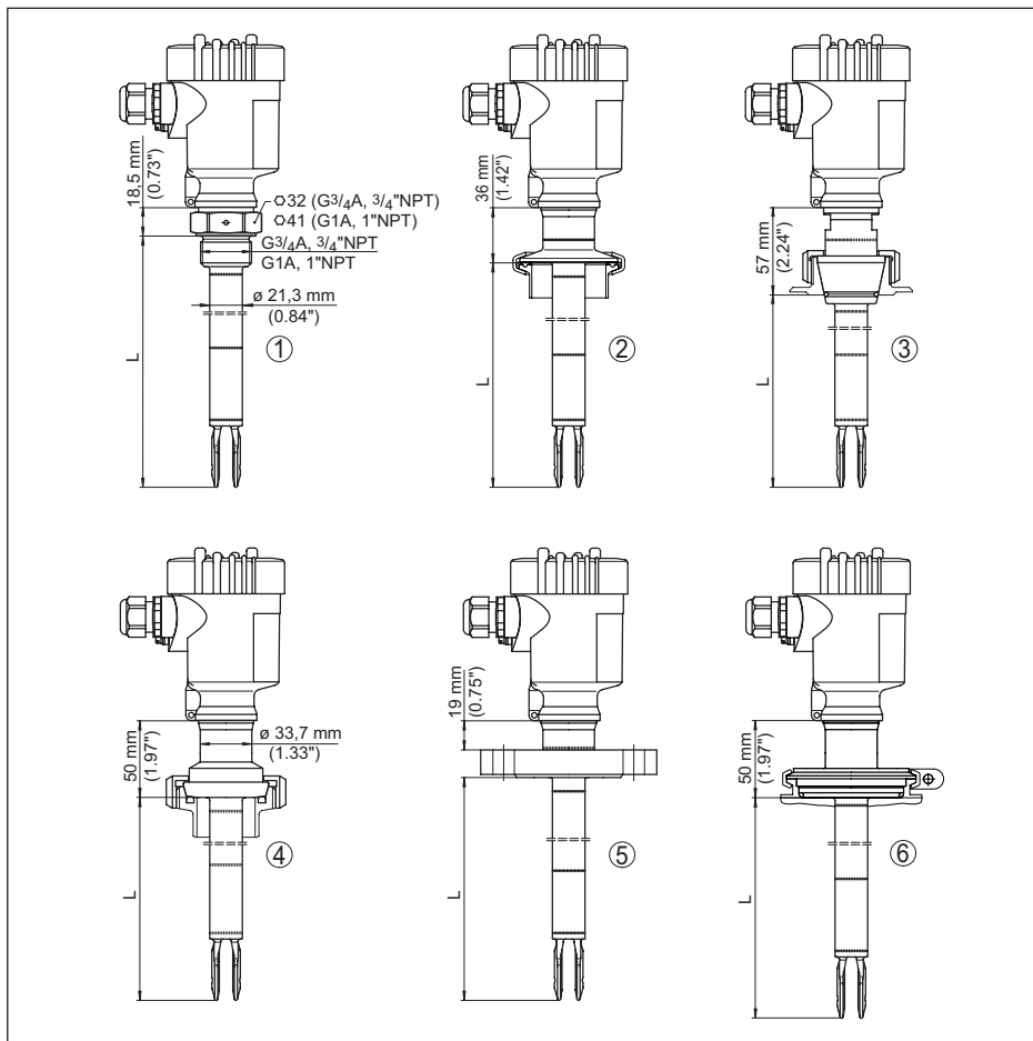
Fig. 38: VEGASWING 63
