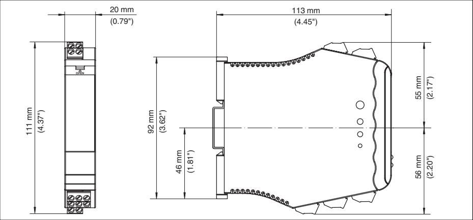
Fig. 54: Dimensions VEGATOR 122
