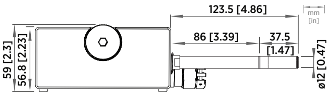
HMP371 dimensions
