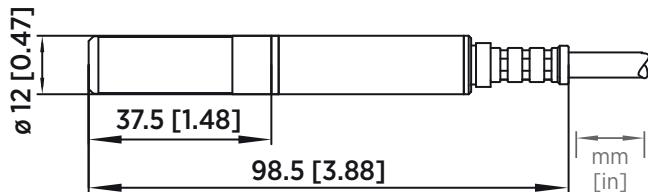
HMP373 dimensions
